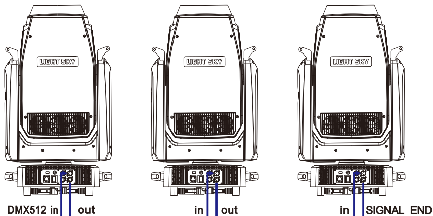
DMX-input
